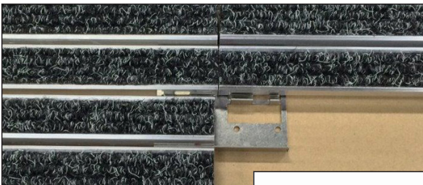
Koppling (connector) som placeras i skarvar och förenar mattdelarna i brunnen. I bilden ovan är 3 mattdelar fixerade i kopplingen.
